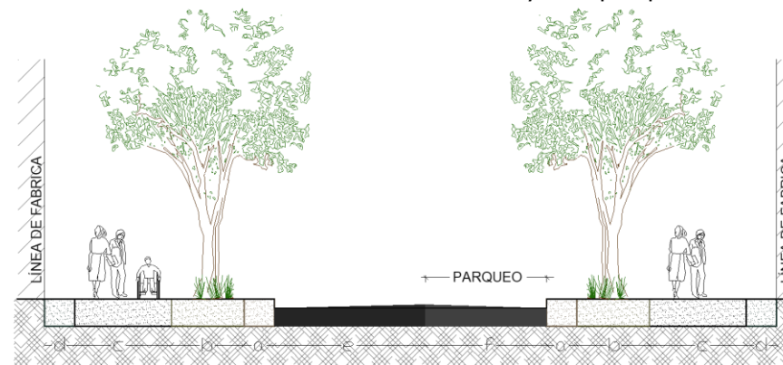
Gráfico 19: calle L2, perfil tipo
